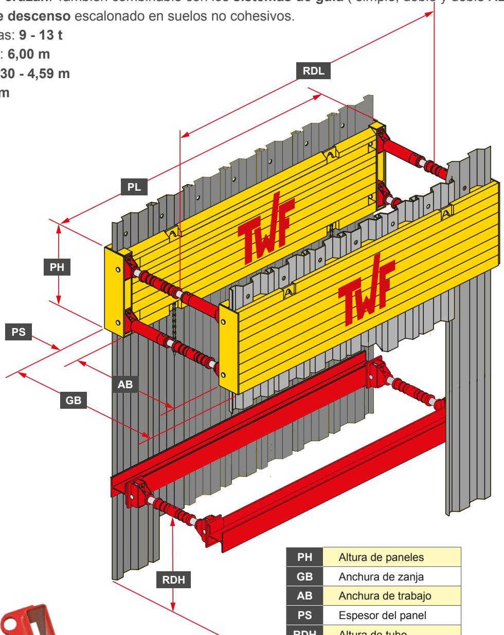
► Codal con cabezal para vigas HEB
